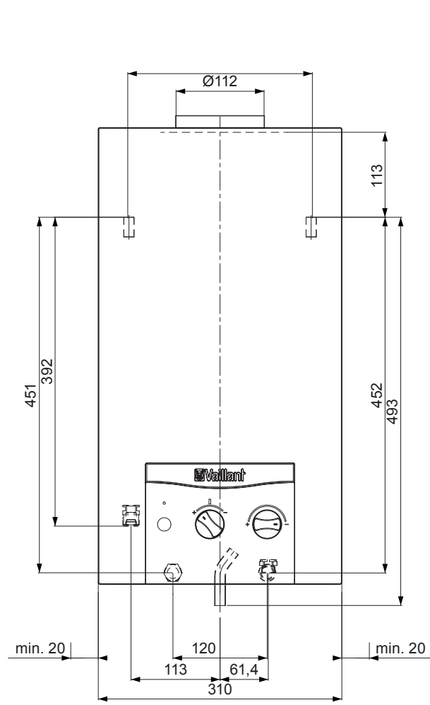
AtmoMAG mini 114/LT 11
