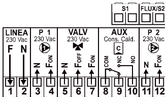
Fig. 1 Aspetto esterno e Schema dei collegamenti elettrici
