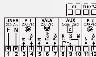
Fig. 1 Aspetto esterno e Schema dei collegamenti elettrici
